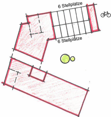
Stellplätze Grundriss EG
